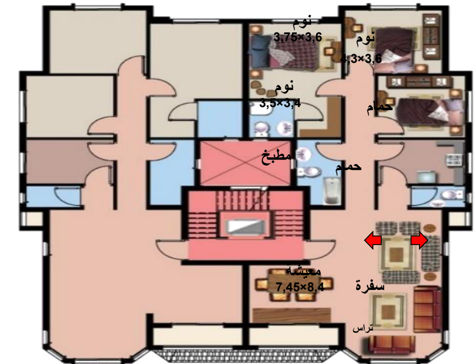
مسقط أفقى الدور المتكرر والاخير
